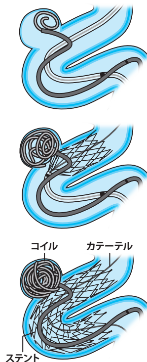
図2 カテーテルによる脳血管内コイル術
